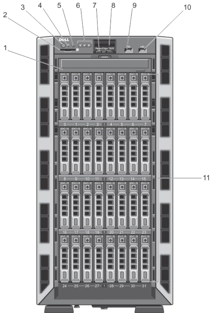
그림 1. 전면 패널 구조 및 표시등—2.5인치 하드 드라이브 새시
