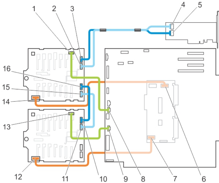
그림 61. 케이블 연결—단일 PERC 카드를 포함하는 2.5인치 (x32) SAS/SATA 후면판
