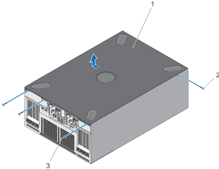
그림 62. 시스템 왼쪽 덮개 분리 및 설치
