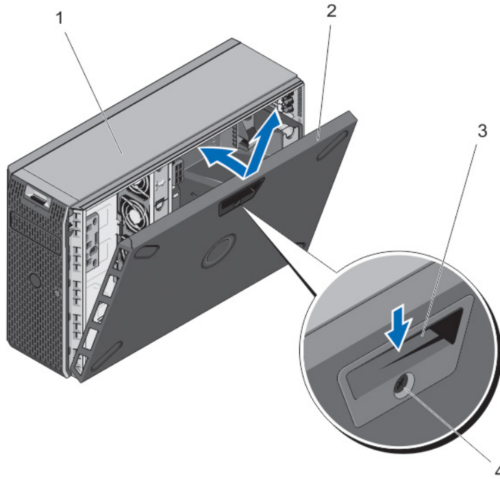
그림 13. 시스템 열기 및 닫기
