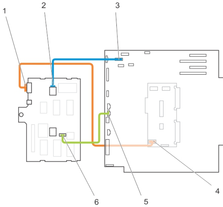
그림 47. 케이블 연결—3.5인치 (x8) SAS/SATA 후면판
