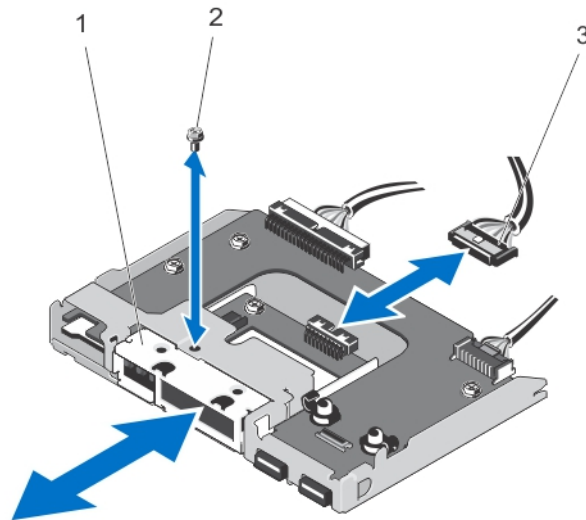
그림 67. 타워 모드에서의 LCD 모듈 분리 및 설치
