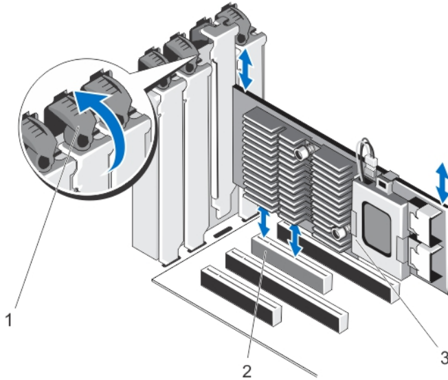
그림 31. 확장 카드 분리 및 설치
