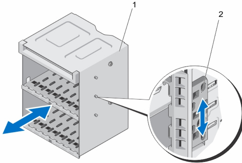
그림 19. 플렉스 베이 분리 및 설치
