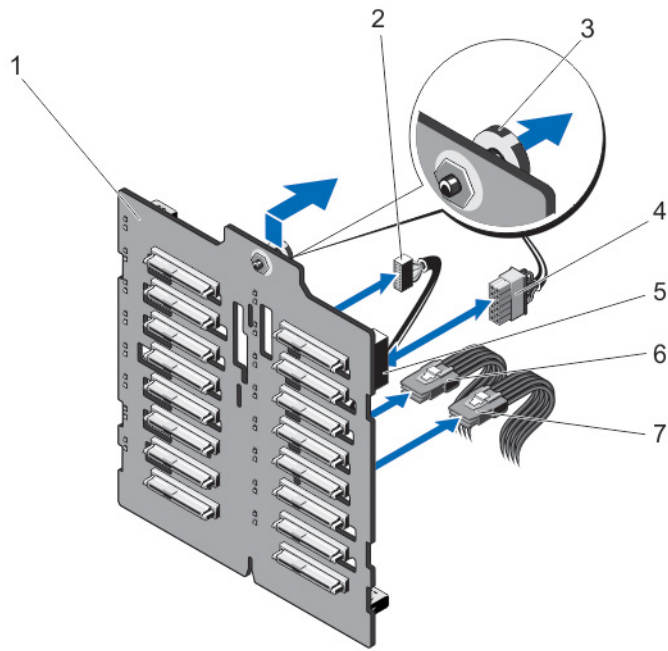
그림 54 . 2.5인치 (x16) SAS/SATA 후면판 분리 및 설치
