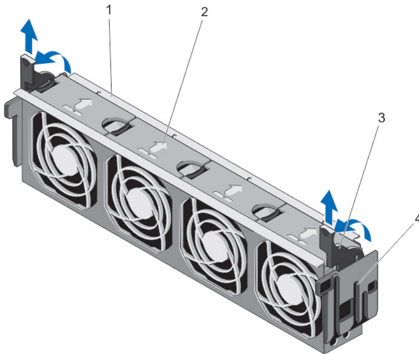
그림 28. 냉각 팬 조립품 분리 및 장착
