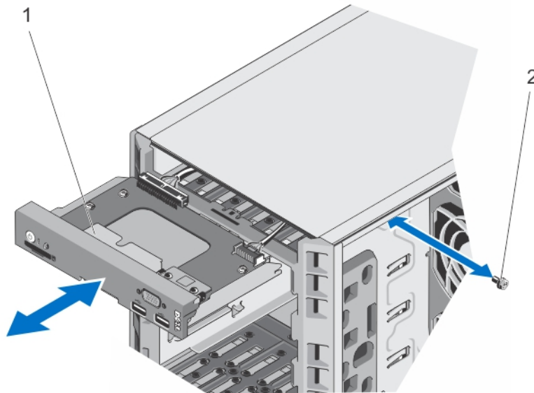
그림 64. 콘솔 모듈 분리 및 설치—랙 모드
