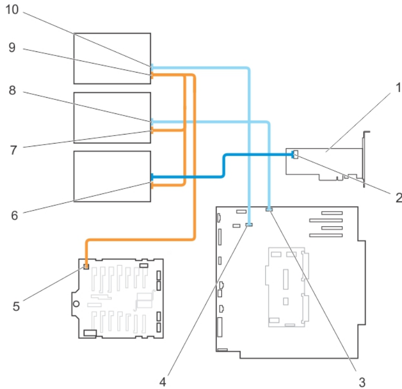
그림 26. 케이블 연결—광학 드라이브 및 테이프 드라이브
