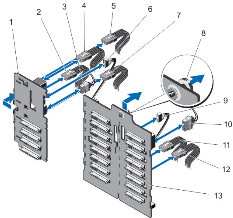
그림 56. 2.5인치 (x16) 및 2.5인치 (x4) SAS/SATA 후면판의 분리 및 설치
