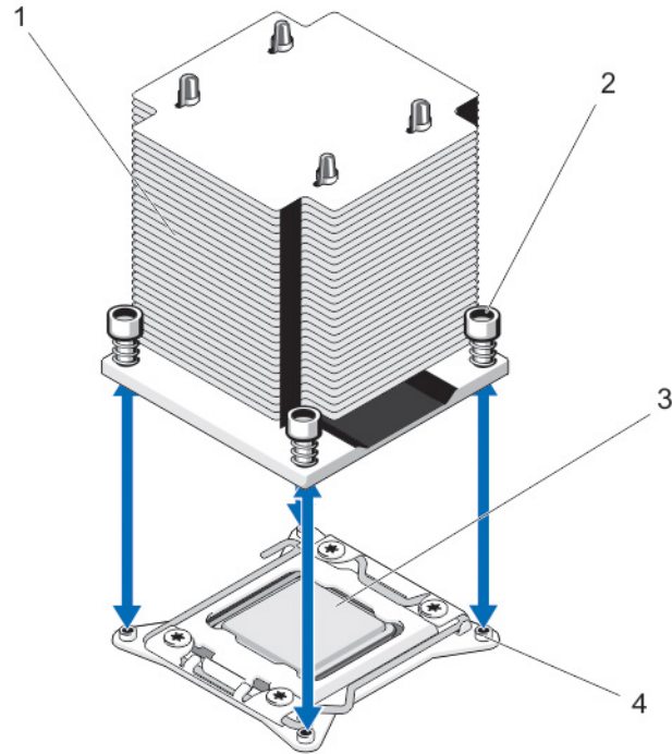
그림 35. 프로세서 분리 및 설치
