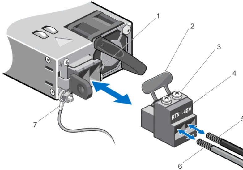
그림 40. DC 입력 전선 조립
