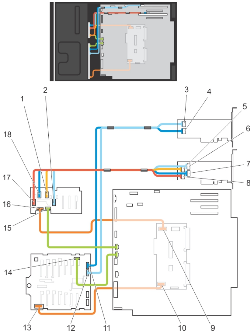
그림 57. 케이블 연결—2.5인치 (x16) 및 2.5인치 (x4) SAS/SATA 후면판
