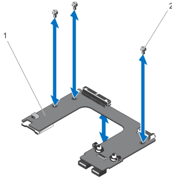
그림 66. 제어판 보드 분리 및 설치
