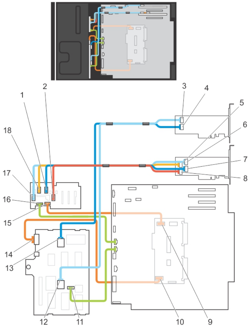
그림 51. 케이블 연결—3.5인치 (x8) 및 2.5인치 (x4) SAS/SATA 후면판
