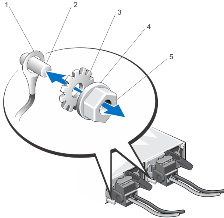
그림 39. 안전 접지선 조립 및 연결
