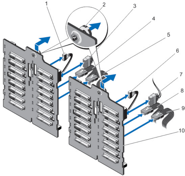
그림 58 . PERC 카드 2개를 포함하는 2.5인치 (x32) SAS/SATA 후면판의 분리 및 설치
