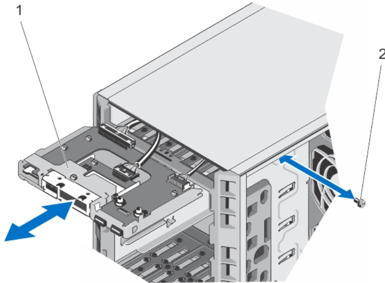
그림 63. 제어판 분리 및 설치—타워 모드
