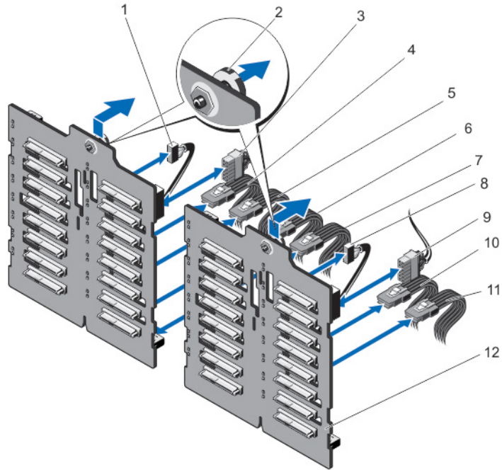
그림 60. 단일 PERC 카드를 포함하는 2.5인치 (x32) SAS/SATA 후면판의 분리 및 설치
