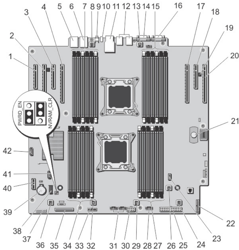
그림 71. 시스템 보드 점퍼 및 커넥터
