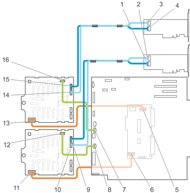
그림 59. 케이블 연결—PERC 카드 2개를 포함하는 2.5인치 (x32) SAS/SATA 후면판
