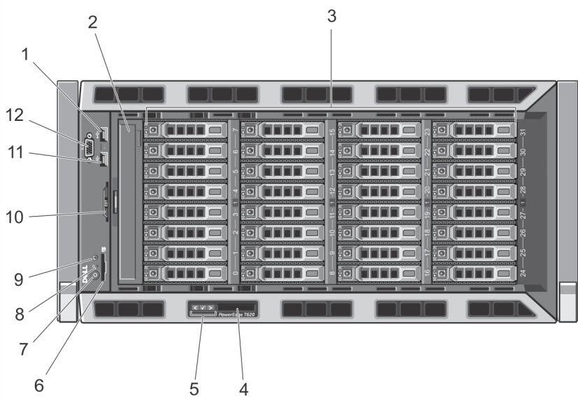
그림 3. 전면 패널 구조 및 표시등—2.5인치 하드 드라이브 새시
