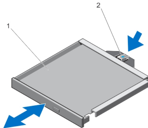
그림 24. 슬림 광학 드라이브 보호물 분리 및 설치
