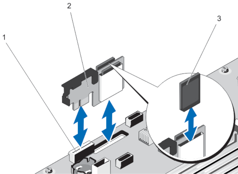
그림 34. 내부 이중 SD 모듈 분리 및 설치
