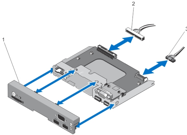
그림 65. 콘솔 모듈에서 콘솔 분리 및 설치—랙 모드
