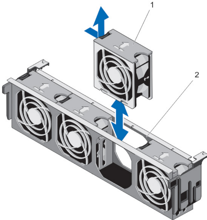
그림 27. 냉각 팬 조립품에서 냉각 팬 분리 및 설치
