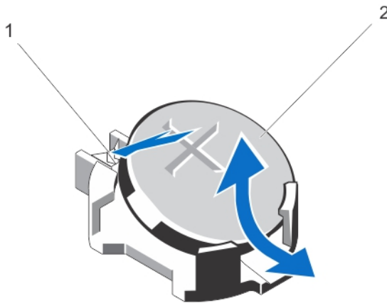
그림 44. 시스템 전지 분리 및 설치
