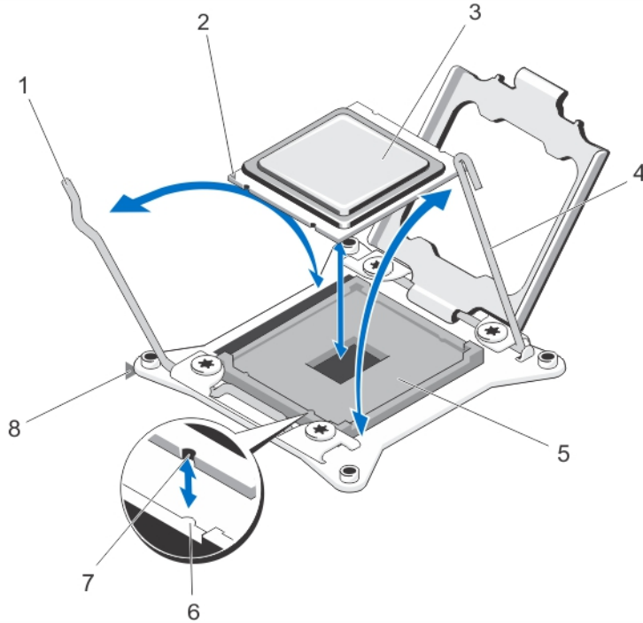
그림 37. 프로세서 분리 및 설치
