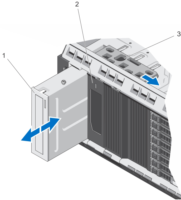
그림 25. 광학 드라이브 또는 테이프 드라이브 분리 및 설치
