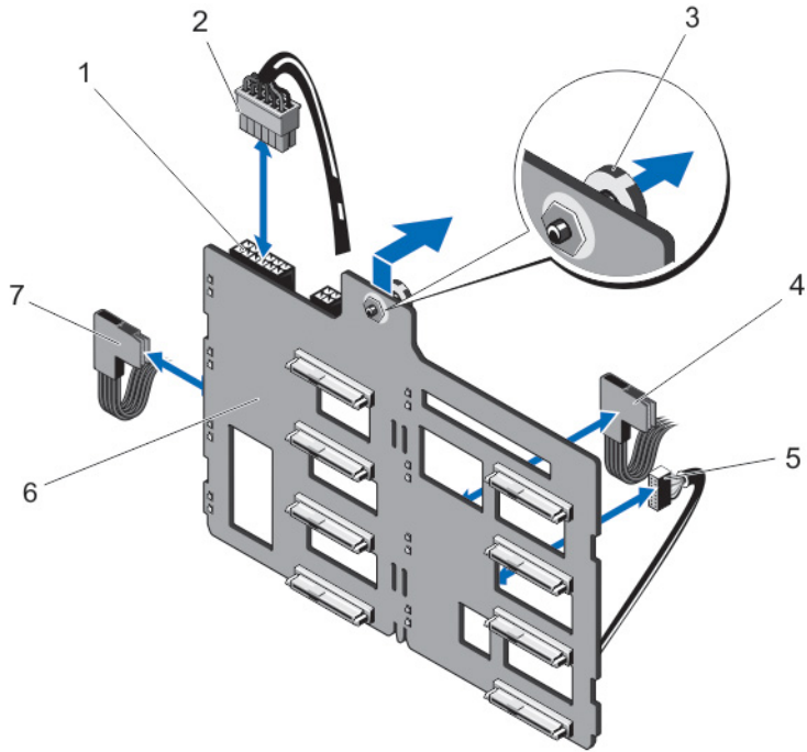
그림 48 . 단일 PERC 카드를 포함하는 3.5인치 (x8) SAS/SATA 후면판의 분리 및 설치
