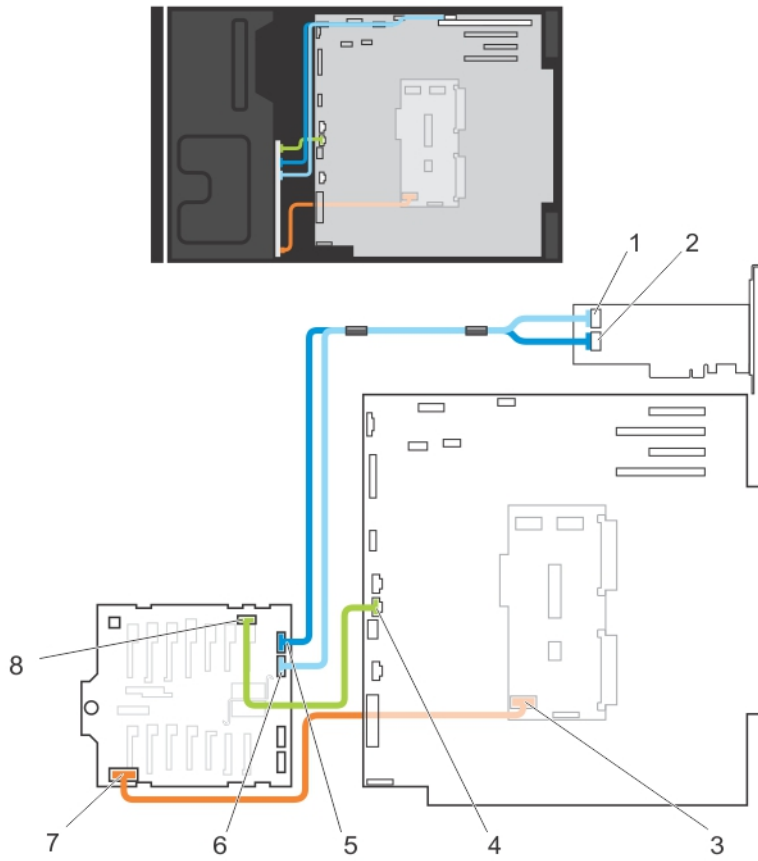
그림 55. 케이블 연결—2.5인치 (x16) SAS/SATA 후면판
