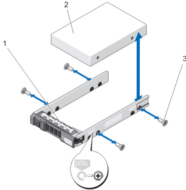
그림 23. 하드 드라이브 캐리어에서 하드 드라이브 분리 및 설치
