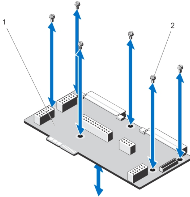
1. 배전 보드
