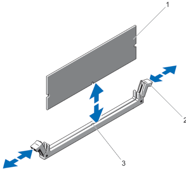
그림 18. 메모리 모듈 분리 및 설치
