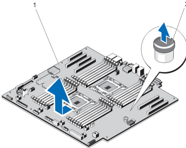
그림 70. 시스템 보드 분리
