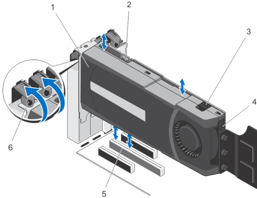
그림 32. GPU 카드 분리 및 설치
