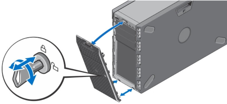
그림 10. 전면 베젤 설치 및 분리
