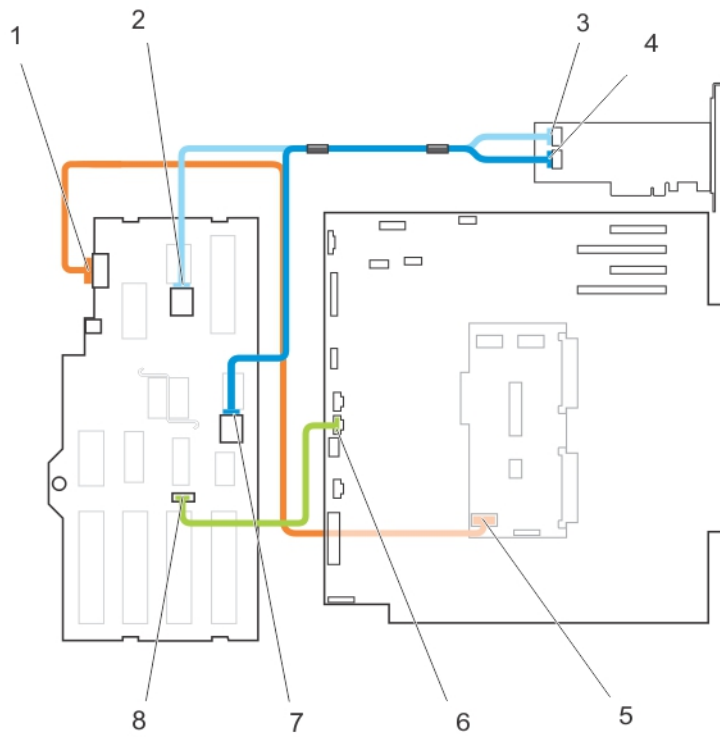
그림 53. 케이블 연결—3.5인치 (x12) SAS/SATA 후면판
