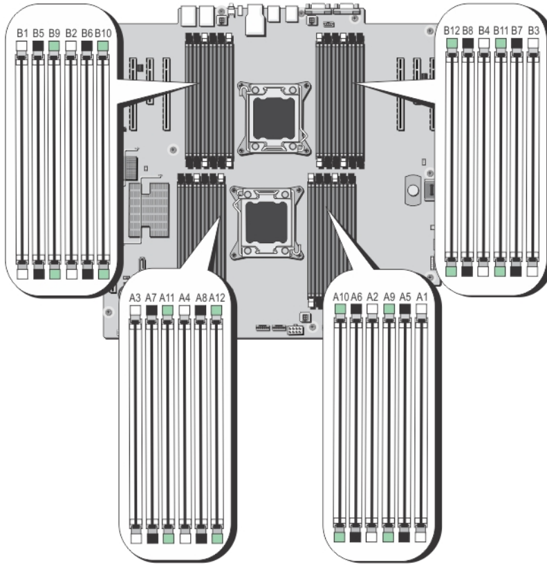
그림 17. 메모리 소켓 위치
