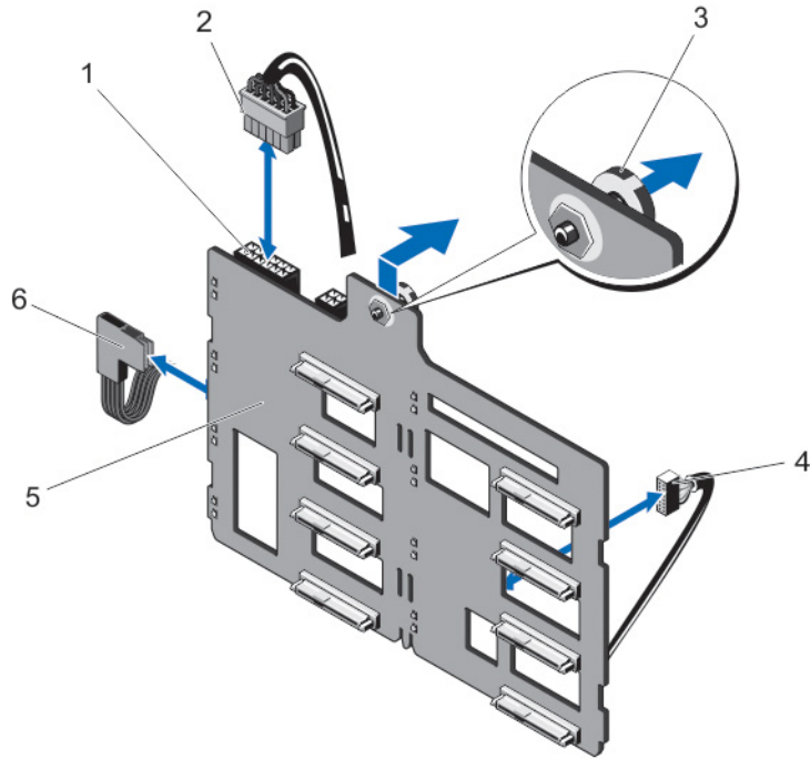
그림 46 . 3.5인치 (x8) SAS/SATA 후면판
