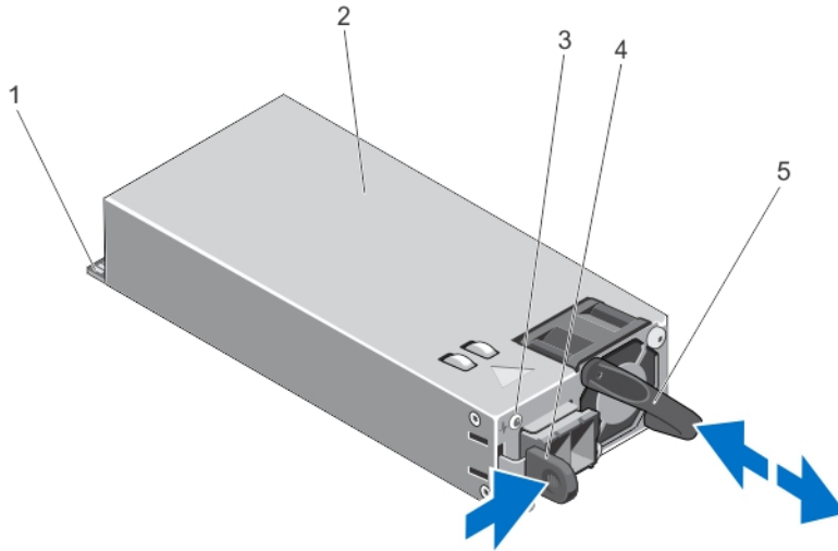
그림 41. DC 전원 공급 장치 분리 및 설치
