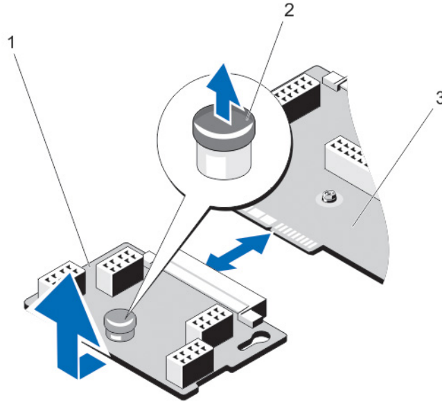
그림 43. 전원 접속기 보드 분리 및 설치
